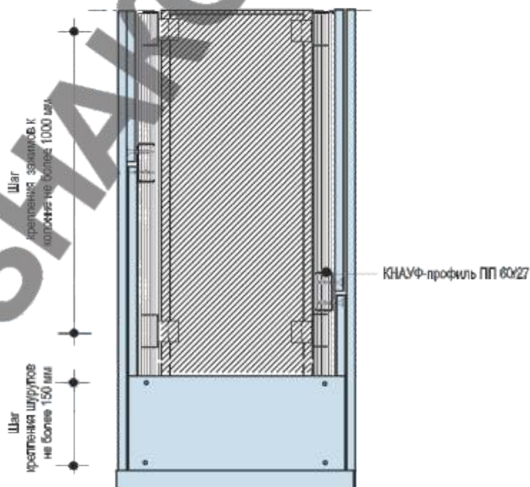
Рис. 2. Конструктивная схема двухслойной облицовки листами ГВЛ ГОСТ Р 51829-2001 толщиной по 12,5 мм каждый ( 2 \times 12,5 = 25 мм).
